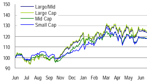
STOXX EuroZone
