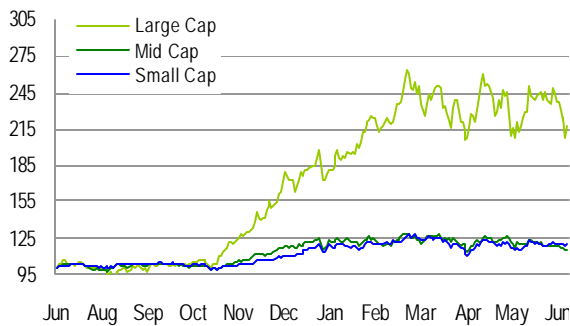
STOXX Nordic
