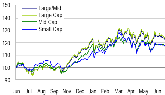
STOXX
